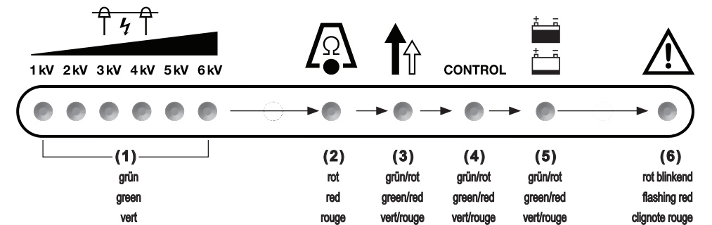
Fig. 3 / LED-Test
